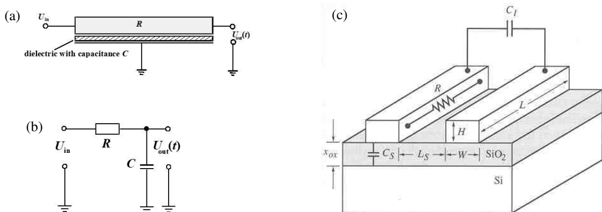
Abbildung 1: (a) zeigt den Längsschnitt einer Verbindungsleitung, welche vom Si-Substrat durch ein Dielektrikum ( SiO_2 ) getrennt ist. (b) „Standard“-RC-Ersatzschaltbild und (c) dreidimensionale Darstellung der Verbindungsleitung mit Widerstand R und den resultierenden Kapazitäten: C_S = Kapazität Leitung/Substrat, C_I = Kapazität Leitung/Leitung.
