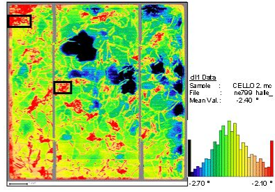
Kurzschlußstrom: Phase
